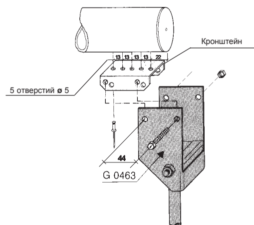
Установка G 0463 стрелу круглого сечения
