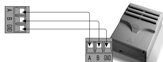
RBM84: система контроля доступа.
