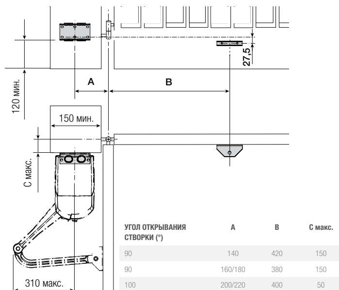
УСТАНОВОЧНЫЕ РАЗМЕРЫ ПРИВОДА (ММ)
